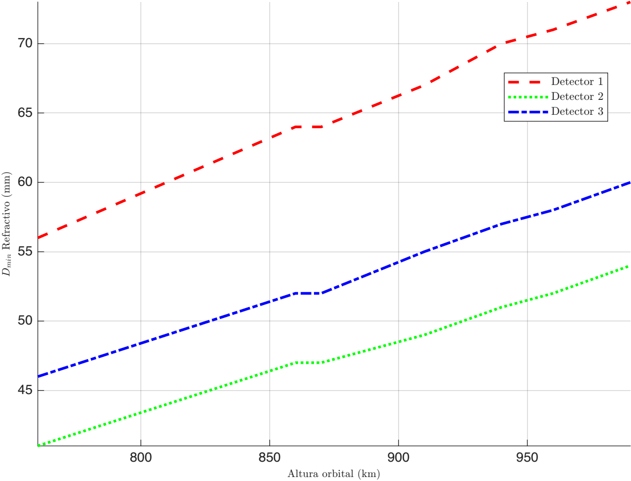
h vs D_{min} - Refractivo - Configuracion: 3 satellite(s), 1 telescopio(s) por satellite
